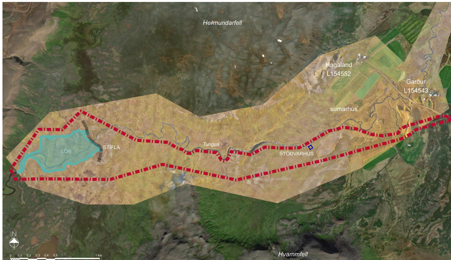
Mynd 2.1 Afmörkun deiliskipulags Tunguárvirkjunar, ásamt legu stöðvarhúss, stíflu og lóns. (Grunnkort: Svarmi 2017 og World Imagery)
