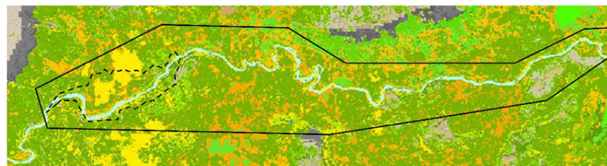
Mynd 2.3 Vistgerðir á skipulagssvæðinu skv. vistgerðakorti NÍ. Gróðurathugunarsvæðið vegna framkvæmdarinnar er afmarkað með svartri línu og fyrirhugað lónstæði er afmarkað með svartri brotlínu. (Kort: Lilja Karlsdóttir 2017)
